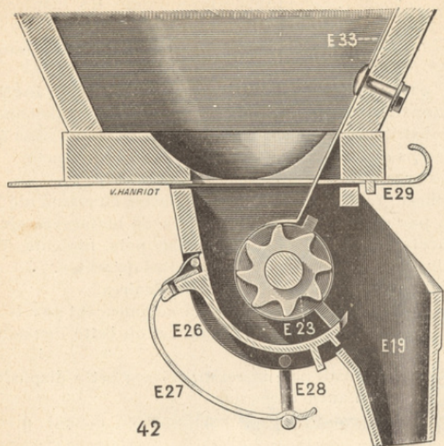
FIG. 4. — Ensemble d'un appareil distributeur à cannelures.
