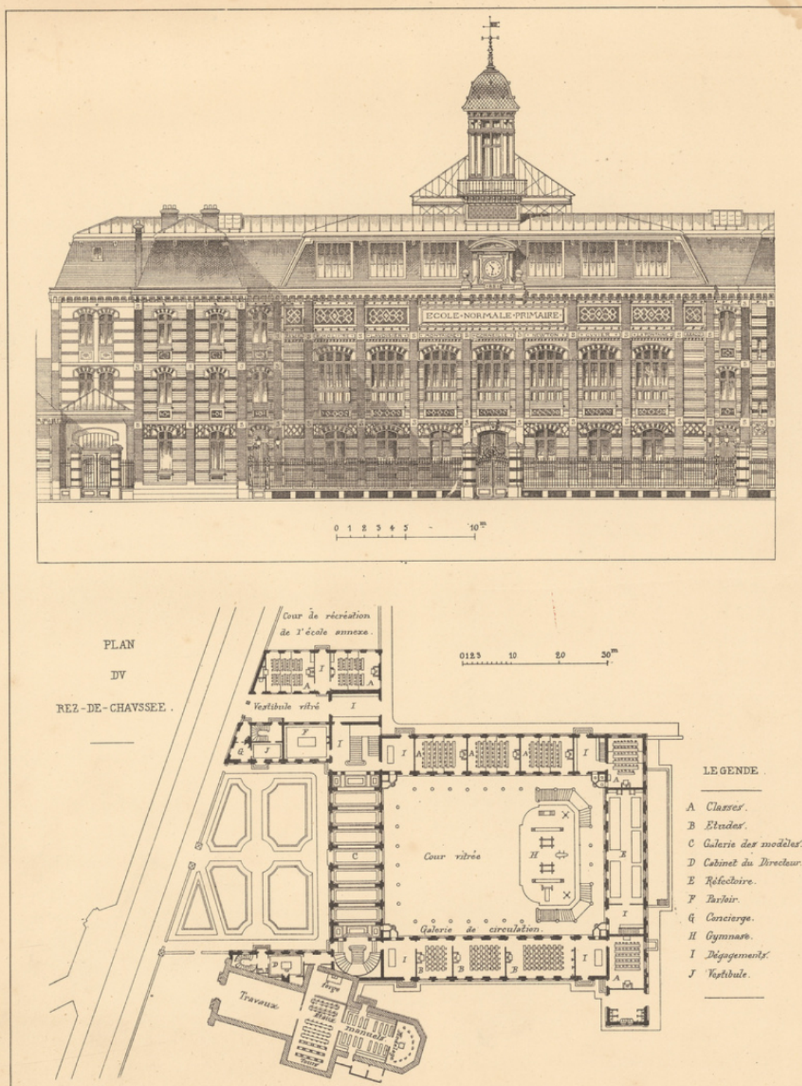
ÉCOLE NORMALE PRIMAIRE A ROUEN — ARCH. M. LEFORT
