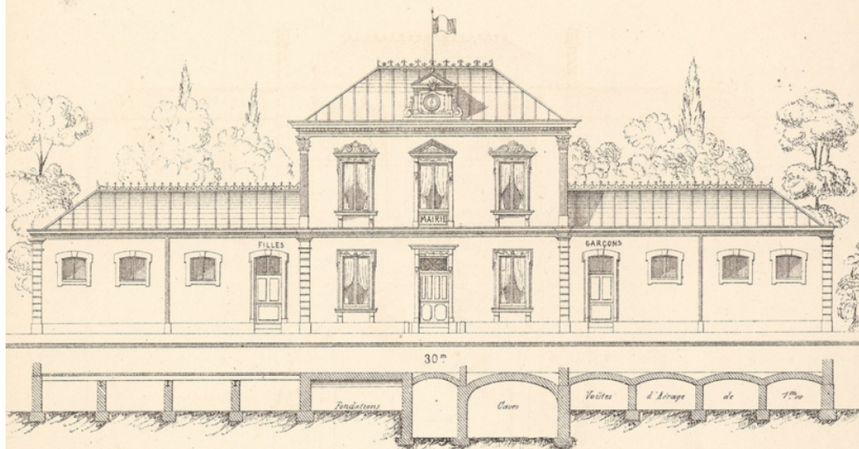
MAIRIE & MAISON D'ÉCOLE TYPE N°1. 18 000 les par G.A. OPPERMANN, Ingénieur-Constructeur. Fig 1. Elevation Générale à 0,007 pour 1 Mètre.
