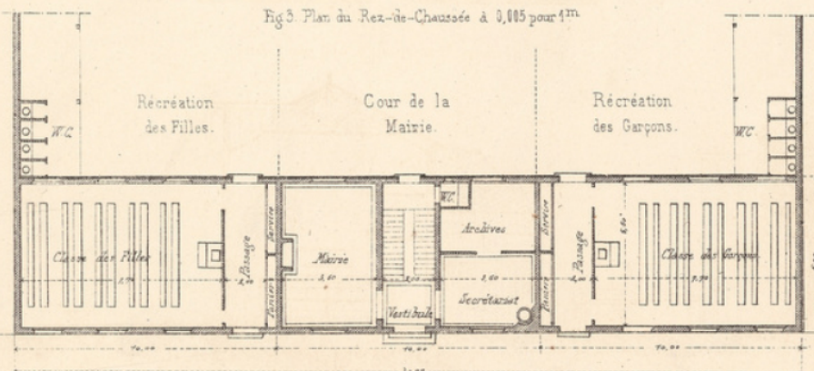
Fig 3. Plan du Rez-de-Chaussée à 0,005 pour 1 m .
