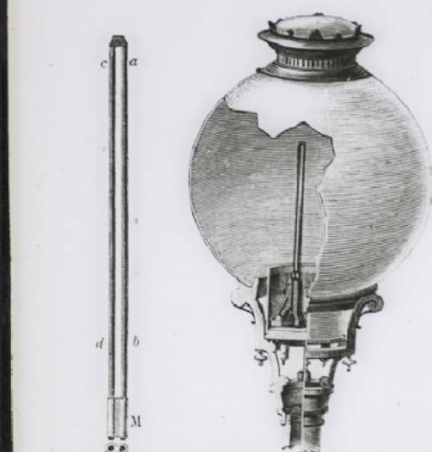
Fig. 310. — Bougie Jablochkoff. Fig. 311. — Globe pour l'éclairage élec- trique par les bougies Jablochkoff.
