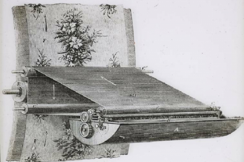
Divers éléments de la machine à imprimer les papiers peints.
