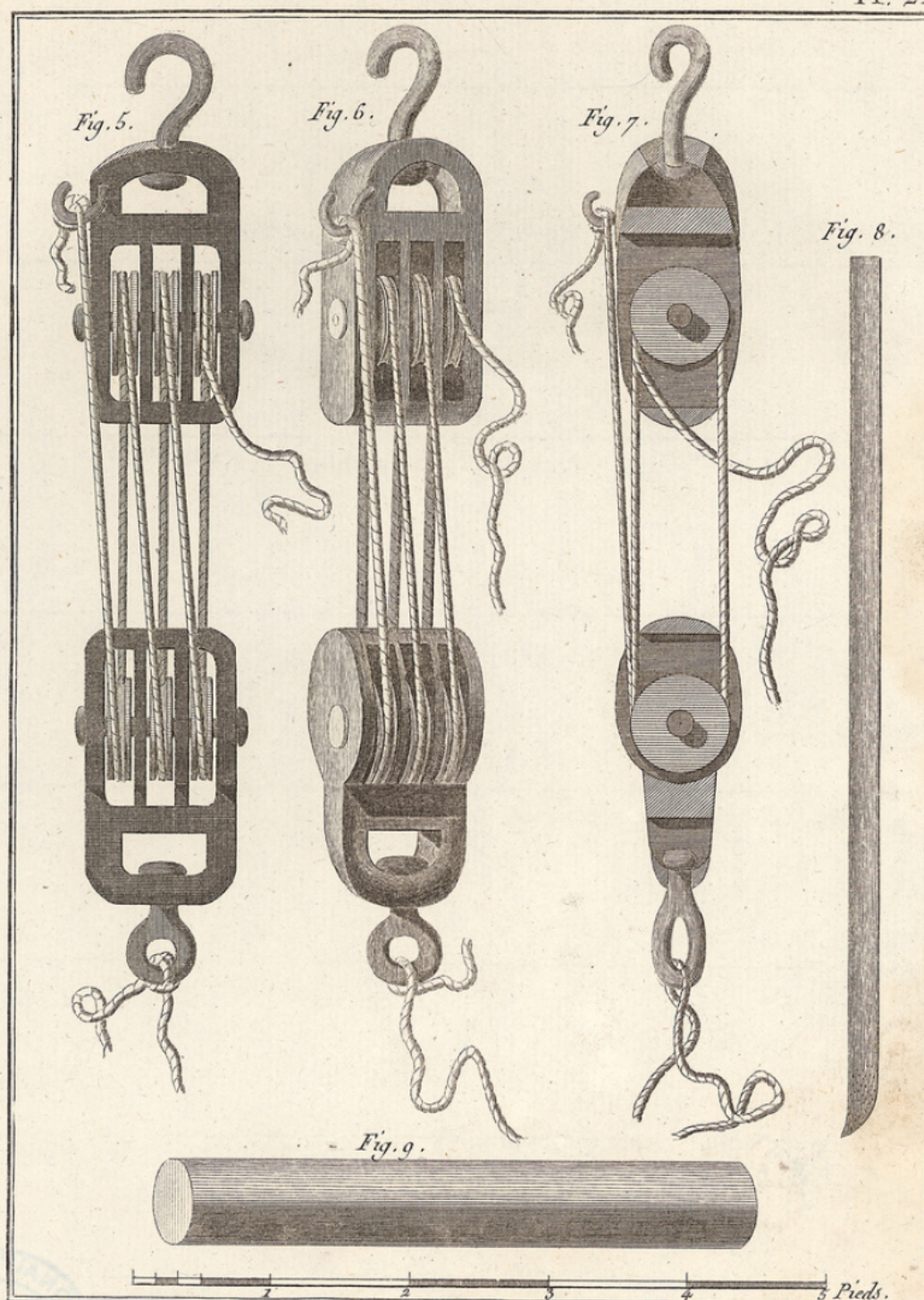
Sculpture, mouffles, Pince et Rouleau pour élever le Marbre. Benard. Dirécit.
