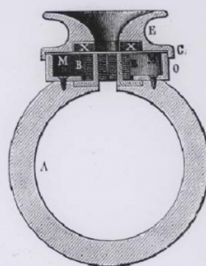
Récepteur Ader. (Perspective et coupe).
