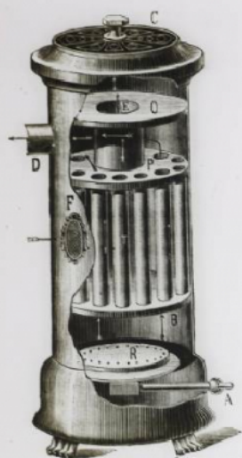
Coupe du calorifère à gaz de M. Wagner.
