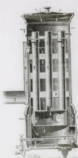
— Coupe du poêle tubulaire de la Compagnie parisienne.
