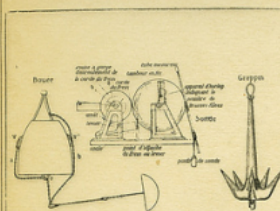
3. — Bouée. — Sonde. — Grappin.
