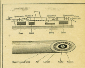
2. — Coupe du navire. — Coupe du câble.
