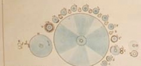
Corte ó sección de una carda
