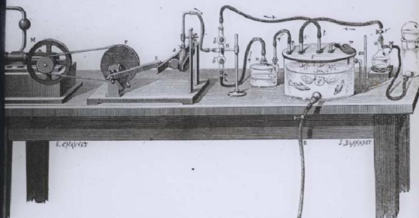
- Appareil de Jolyet et P. Regnard pour l'étude de la respiration chimique des animaux aquatiques.
