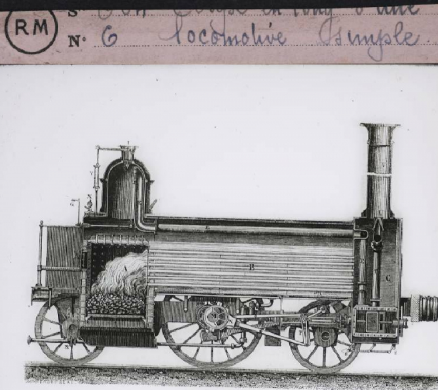
Coupe longitudinale d'une locomotive.
