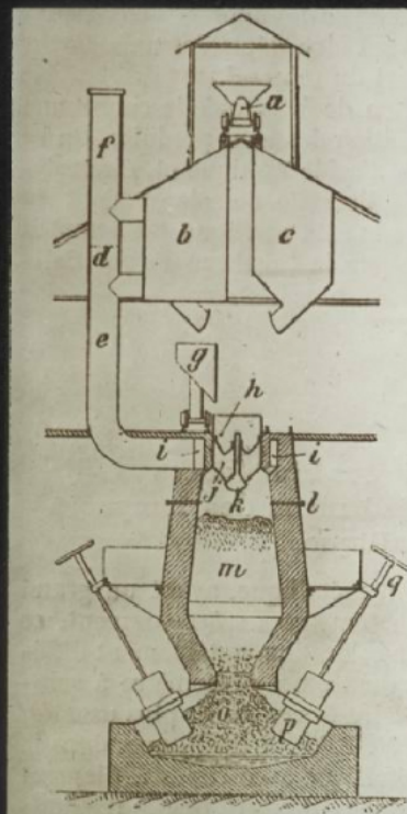
FIG. 15. Ensemble de l'installation du haut fourneau électrique de la Noble Electric Steel Co.
