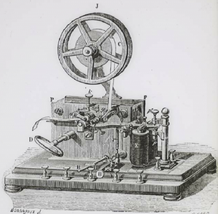
Récepteur de l'appareil Morse à pointe sèche.
