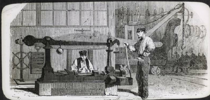
Machine à presser la résine des côtes
