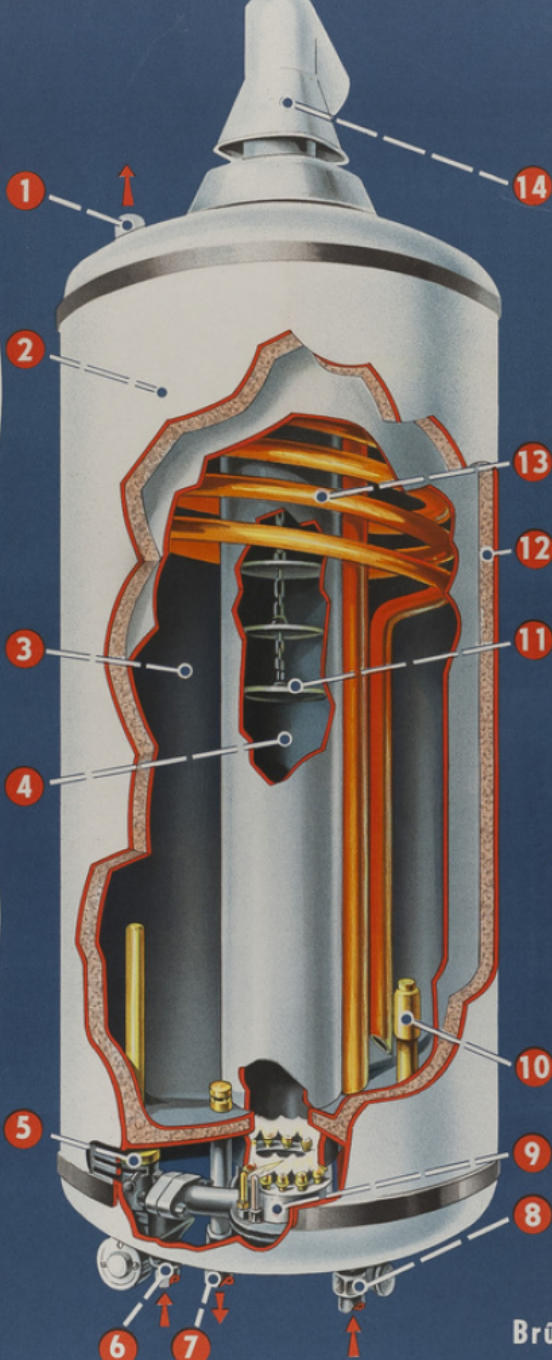
Bloc "eau chaude" d'appartement
