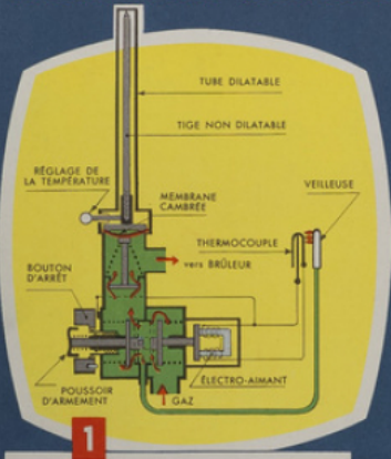
1 Sécurité par thermocouple
