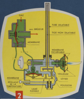
2 Sécurité pneumatique par élément incurvable
