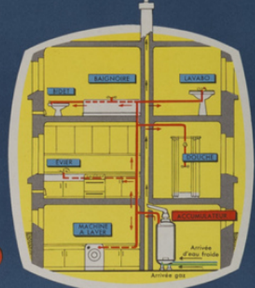
Centrale "eau chaude" d'un pavillon
