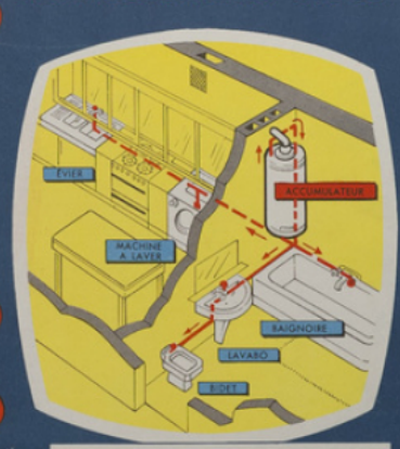
Bloc "eau chaude" d'appartement
