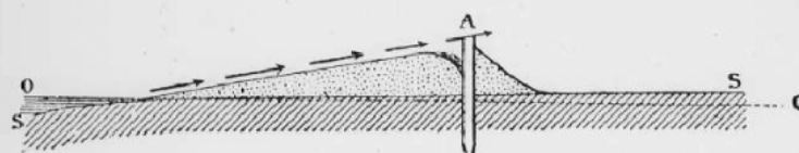
— Formation des dunes. — O. O. niveau de la mer. S. S. sol naturel.
