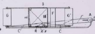
Fig. 2. - Coupe de l'aéroplane suivant X, X.
