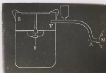
Coupe verticale intérieure du réservoir- régulateur.
