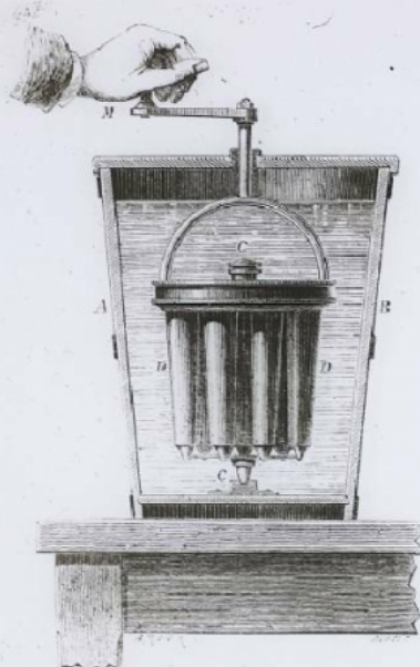
Type général d'une glacière de ménage.
