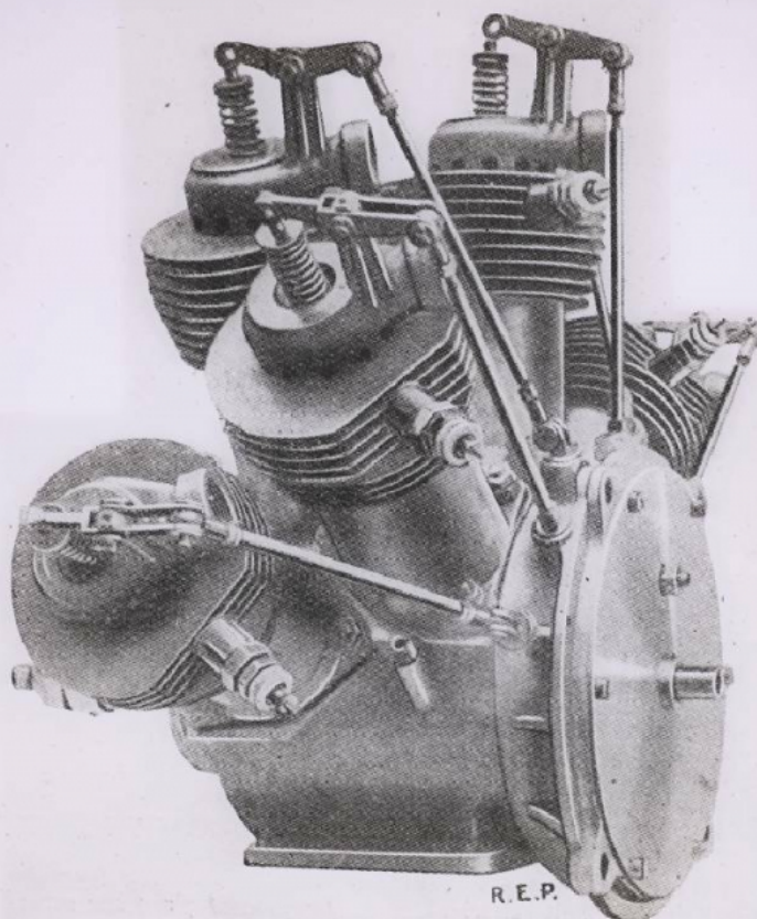
- Le moteur REP vu de côté.
