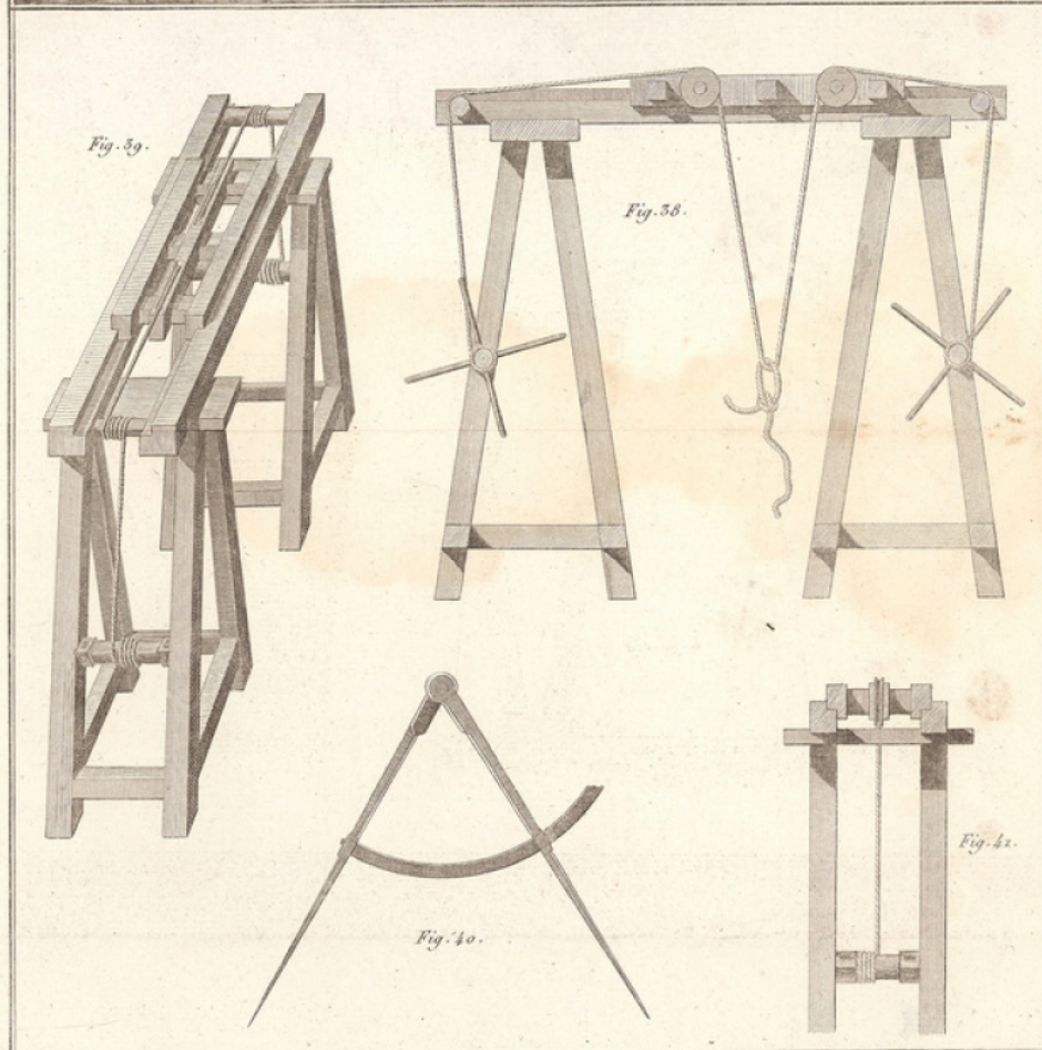
Sculpture, l'opération de traîner le marbre, et machine pour poser les figures à leurs places.
