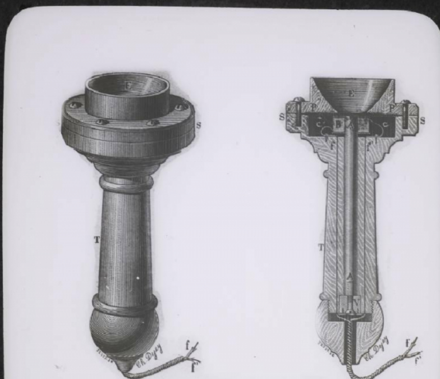
Le téléphone magnétique de Graham Bell (perspective et coupe).
