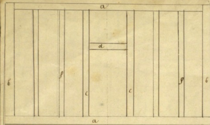
Clouon en charpente a Solliers b Poutres corniers c Poutres d'huberie d Linteau f Montants ou poutres d'emplissage
