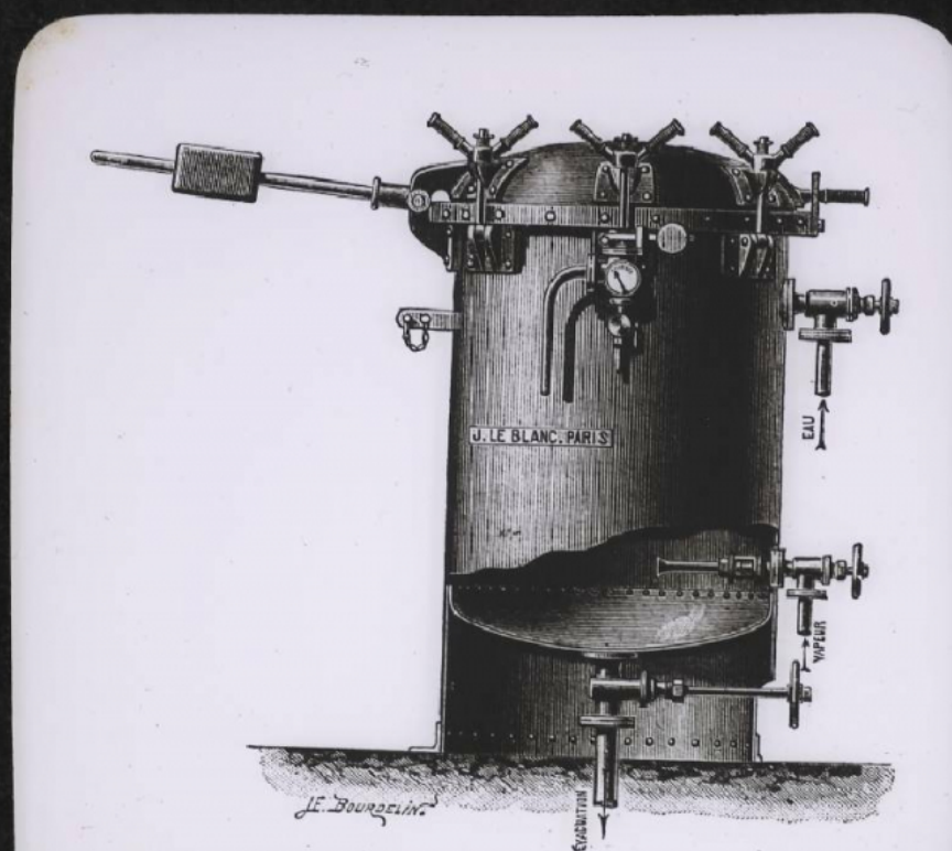
Autoclave pour la désinfection des crachats.
