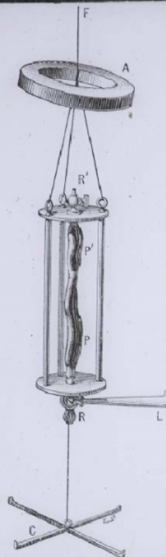
Fig. 172. — Bouteille en caoutchouc de P. Regnard représentée au moment où arrive le pont messager.
