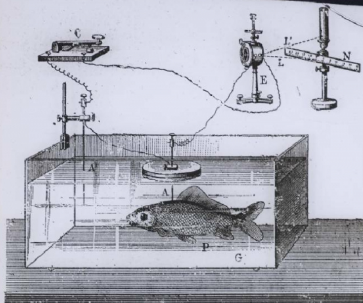
Dispositif destiné à mesurer la différence de température entre l'animal aquatique et l'eau dans laquelle il vit.
