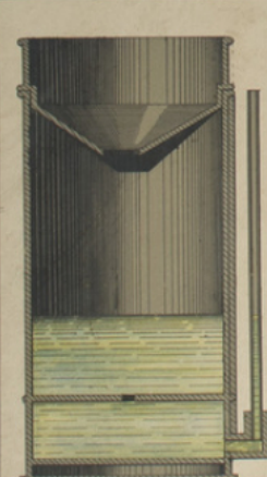
PLUVIOMÈTRE (Coupé) Appareil destiné à mesurer la quantité d'eau de pluie tombée en un lieu.
