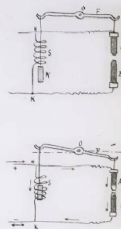
Régulateur pour Lampe à arc
