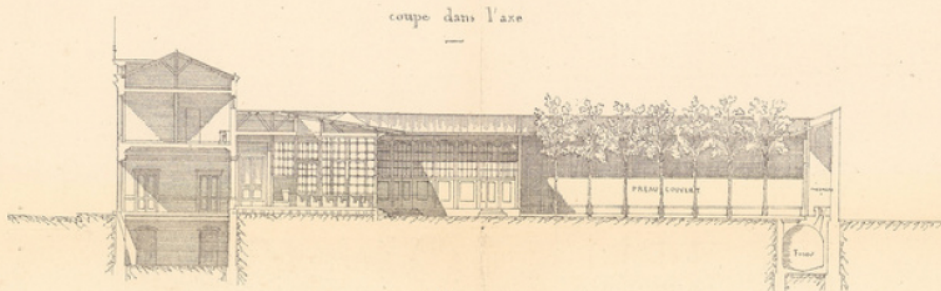
coupe dans l'axe
