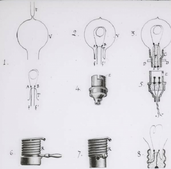
Fabrication d'une Lampe à incandescence Doutilles et Cutols.
