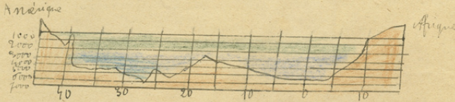
Coupe de l'Atlantique par le tropique du Capricorne
