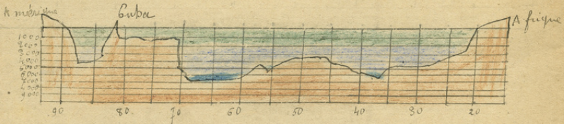
Coupe de l'Atlantique par le tropique du Cancer
