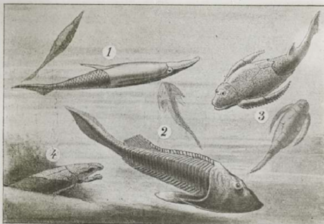
Fig. 110. — Restauration de divers Poissons cuirassés de l'ère primaire 1, Pteraspis ; 2, Cephalaspis ; 3, Pterichthys ; 4, Coccosteus .
