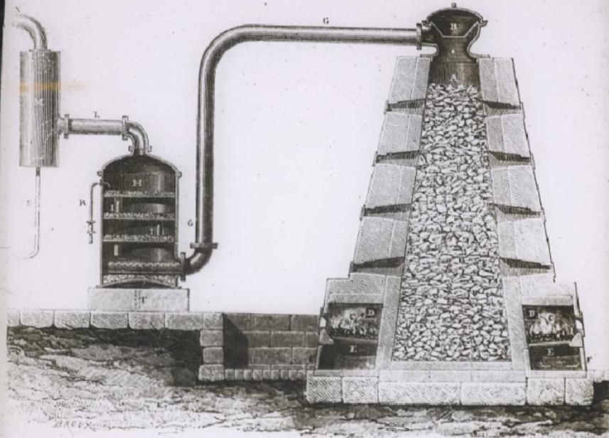
Appareil pour la préparation de la chaux et de l'acide carbonique.
