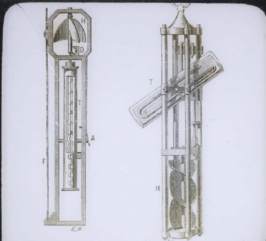
Appareil à retournement de l'amiral Magnaghi.
