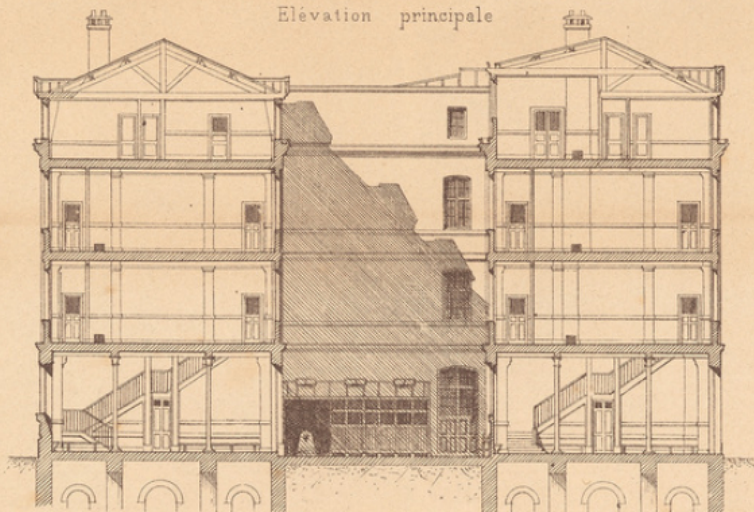
Coupe longitudinale
