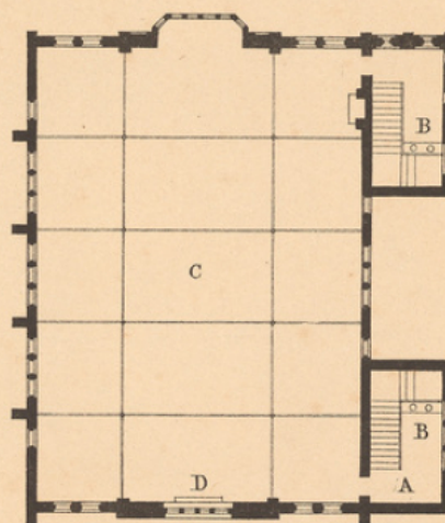
Plan du 1 er Étage.
