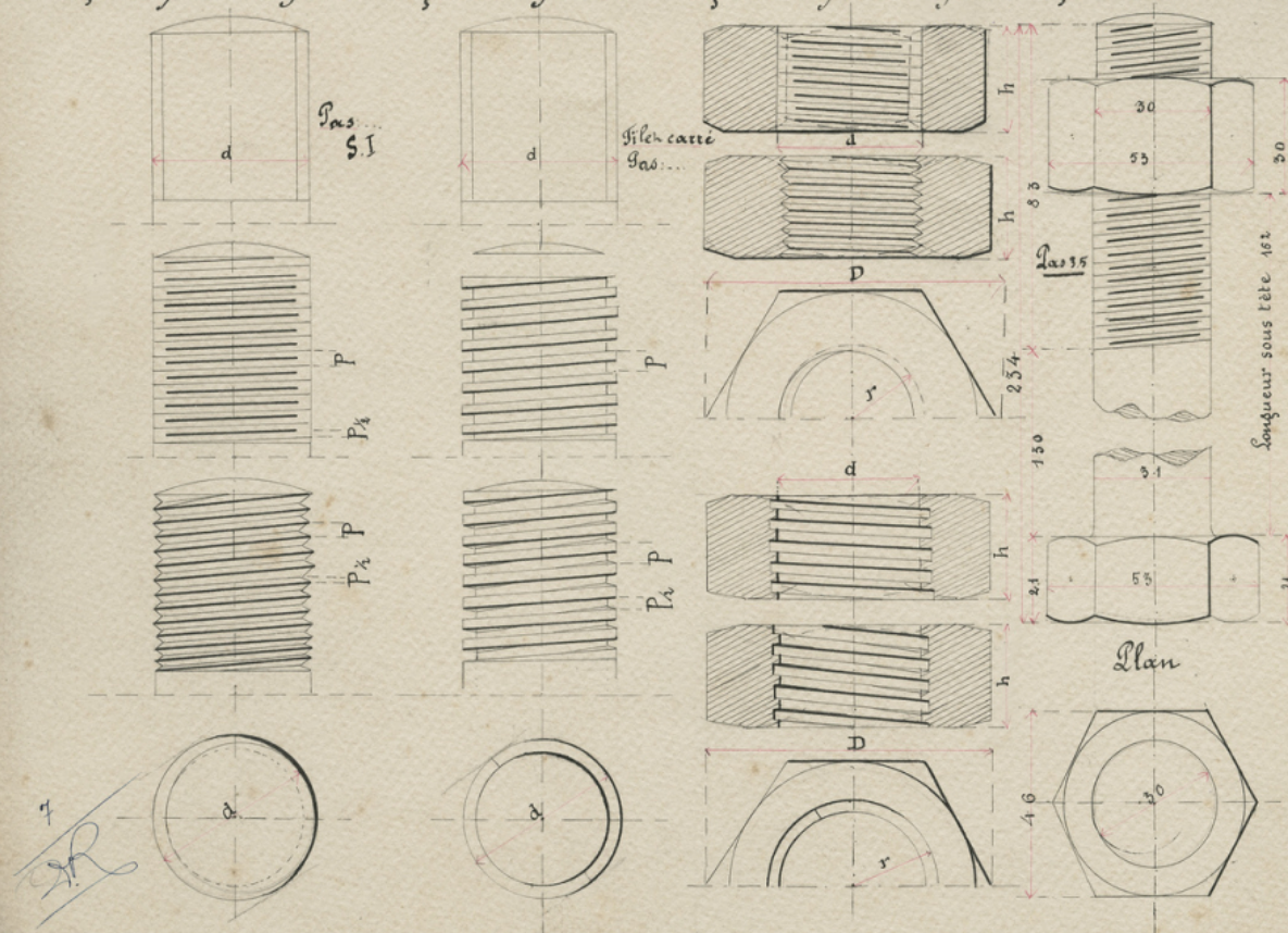
Fig.1. Vis à filets triangulaire Fig.2. Vis à filets carré Fig.3. Ecrou à filets triangulaire Fig.4. Boulon et Ecrou. Ech. \frac{3}{4}
