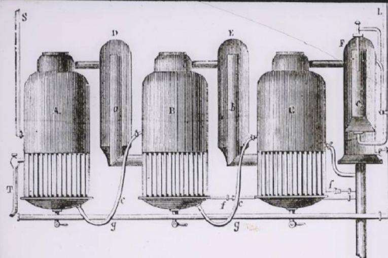
Appareil à triple effet pour l'évaporation des sirops.
