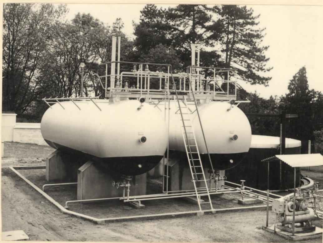
Station de propane d'AVRANCHES qui émet du propane pur et de l'air propané
