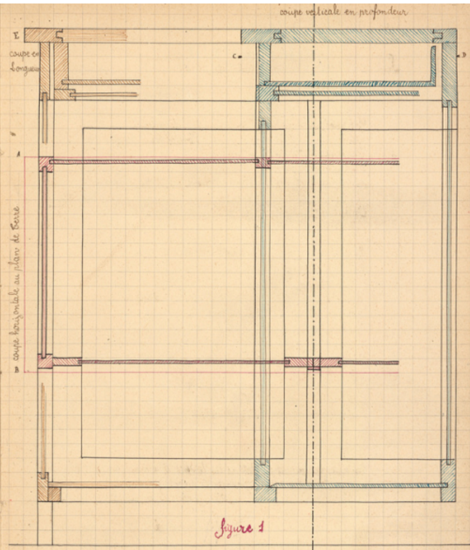
Figure 1 Dessin schématisant la manière d'exprimer les traces de construction d'un meuble (son plan)
