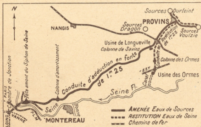
Carte schématique de l'adduction des eaux de la Voulzie et du Durteint, et la restitution en eau de Seine
