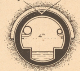
Coupe théorique d'un égout
