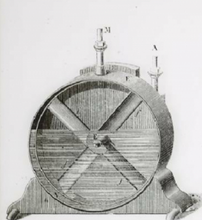
Fig. 100. — Compteur à gaz, coupe de la partie postérieure.
