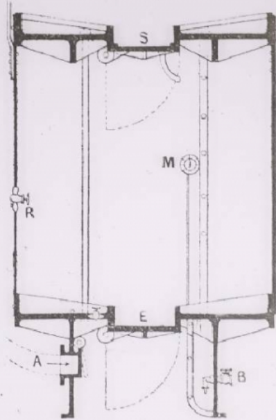
Coupe longitudinale d'une chambre d'air.
