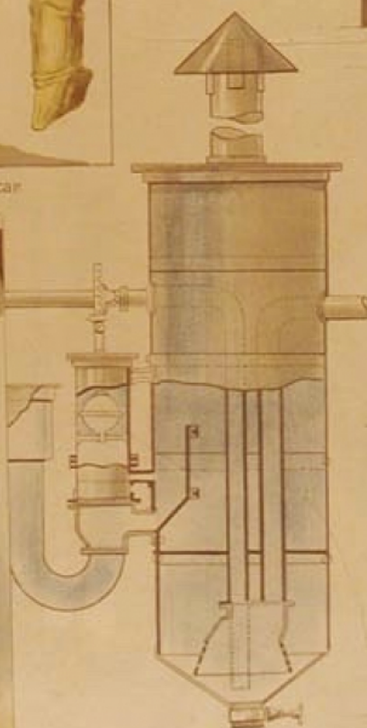
Aparato para la purificación del jugo
