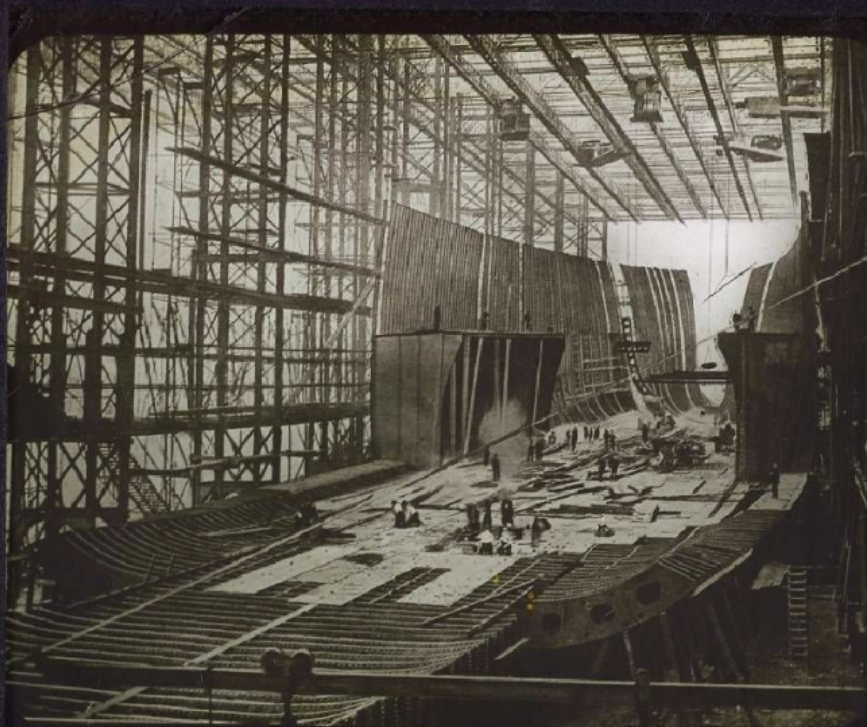
Mise en chantier d'un navire.
