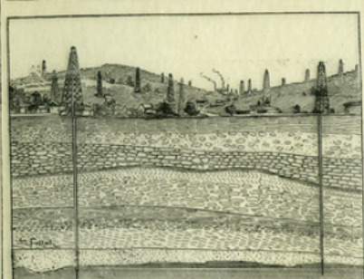
Fig. 1. — Coupe géologique d'un bassin de pétrole en Pennsylvanie.
