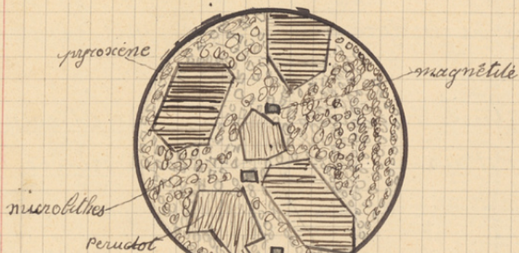
Roche microolithique Basalte vue au microscope
