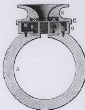
Récepteur Ader. (Perspective et coupe).
